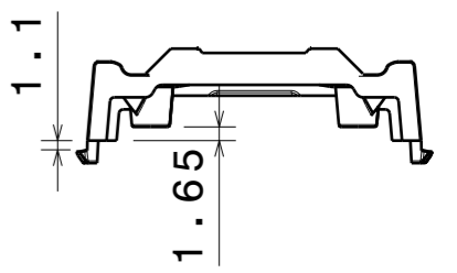
Right View Scale: 1:1
